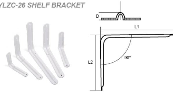
YLZC-26 SHELF BRACKET
